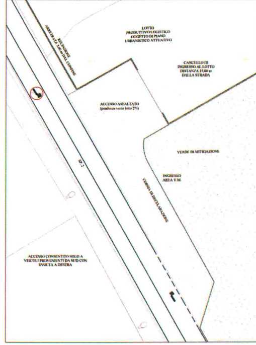
ACCESSO SUD SU SP2
